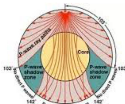
P-wave shadow zone = 103^\circ - 142^\circ
